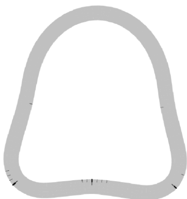
Obr. 4 Lokalizace trhlin (vl. tíha + voda)
