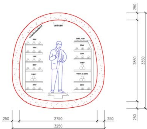
Obr. 2 Příčný řez
